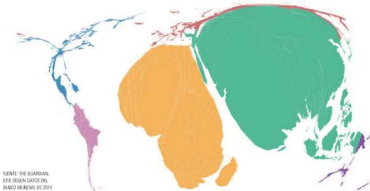
Figura 2. Países que sufren las consecuencias del cambio climático. Fuente: The Guardian 2015 según datos del Banco Mundial de 2013.
