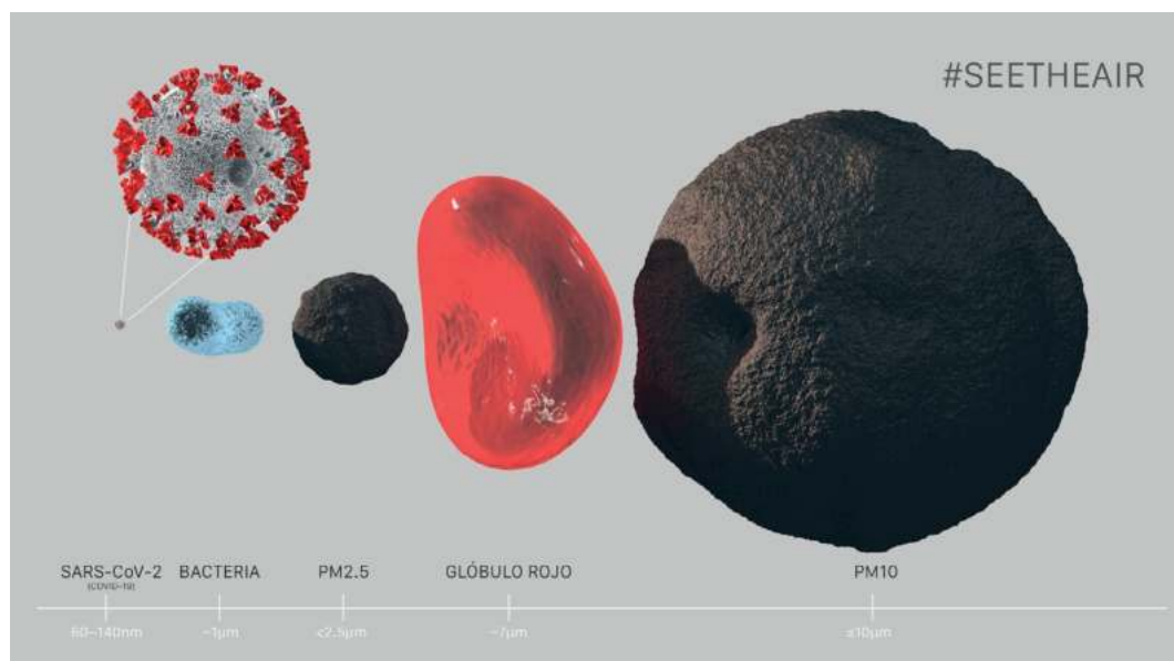
Figura 13. Comparación del tamaño de partículas finas (PM 2.5 ) y gruesas (PM 10 ) con glóbulos rojos, bacterias y virus. Fuente: elaboración por Sotirios Papathanasiou (seetheair.org).
